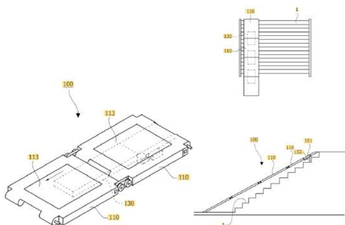
Рисунок 4. «Устройство для лестниц» (Южная Корея)
