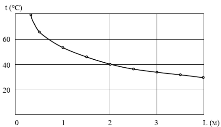
Рисунок 4. Зависимость температуры дыма ( t ) от длины дымопровода ( L )
